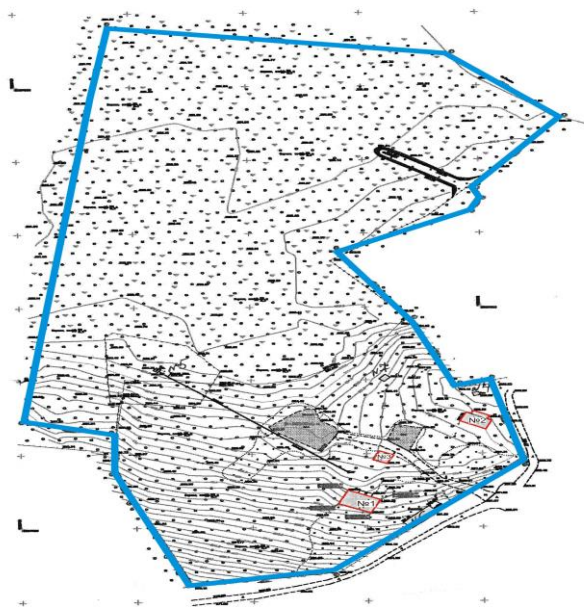
Рисунок 1 – План учебно-геодезической базы «Исеть»
